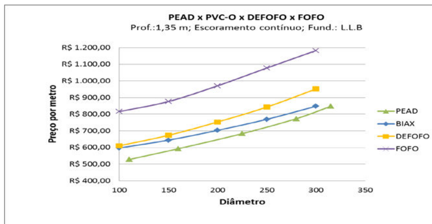
Figura 5: Comparativo com Profundidade de 1,35 m, Escoramento Contínuo e Fundação LLB.
