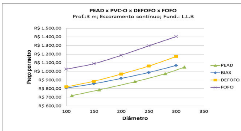
Figura 9: Comparativo com Profundidade de 3m, Escoramento Contínuo e Fundação LLB.
