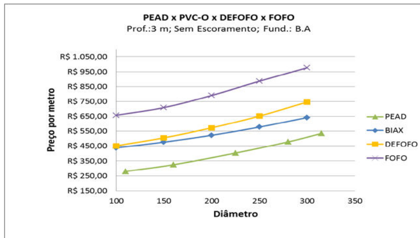
Figura 6: Comparativo com Profundidade de 3,0 m, Sem Escoramento e Fundação Berço de Areia.
