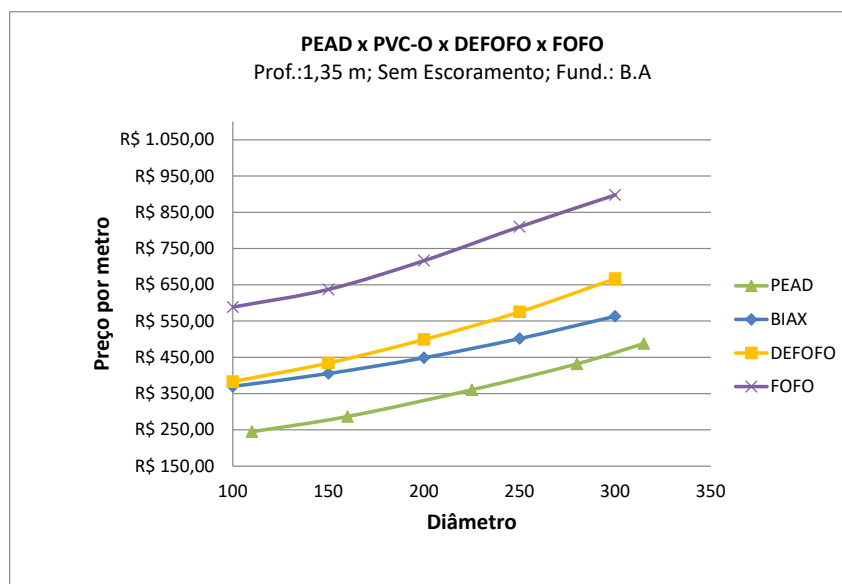
Figura 2: Comparativo com Profundidade de 1,35 m, Sem Escoramento e Berço de Areia.
