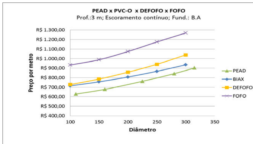
Figura 8: Comparativo com Profundidade de 3m, Escoramento Contínuo e Berço de Areia.
