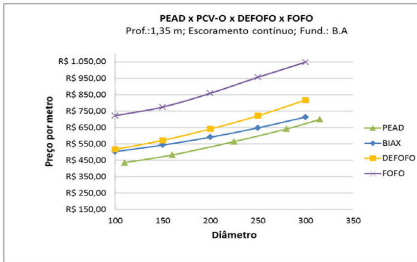
Figura 4: Comparativo com Profundidade de 1,35 m, Escoramento Contínuo e Berço de Areia.
