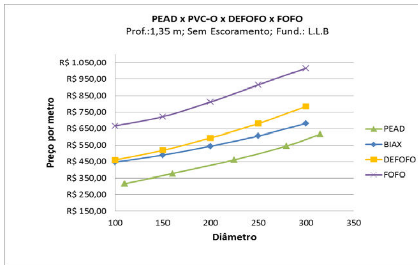
Figura 3: Comparativo com Profundidade de 1,35 m, Sem Escoramento e Fundação LLB.
