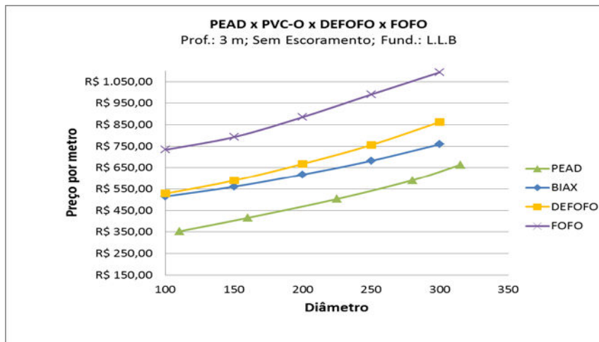
Figura 7: Comparativo com Profundidade de 3m, Sem Escoramento e Fundação LLB.
