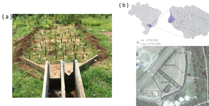
Figura 1 – (a) A bioretenção instalada (pós-adaptações e manutenções); (b) Localização da bioretenção na bacia urbana de São Carlos. Linha pontilhada representa a delimitação de área de drenagem e a TC de bioretenção é identificada pelo polígono em vermelho.
