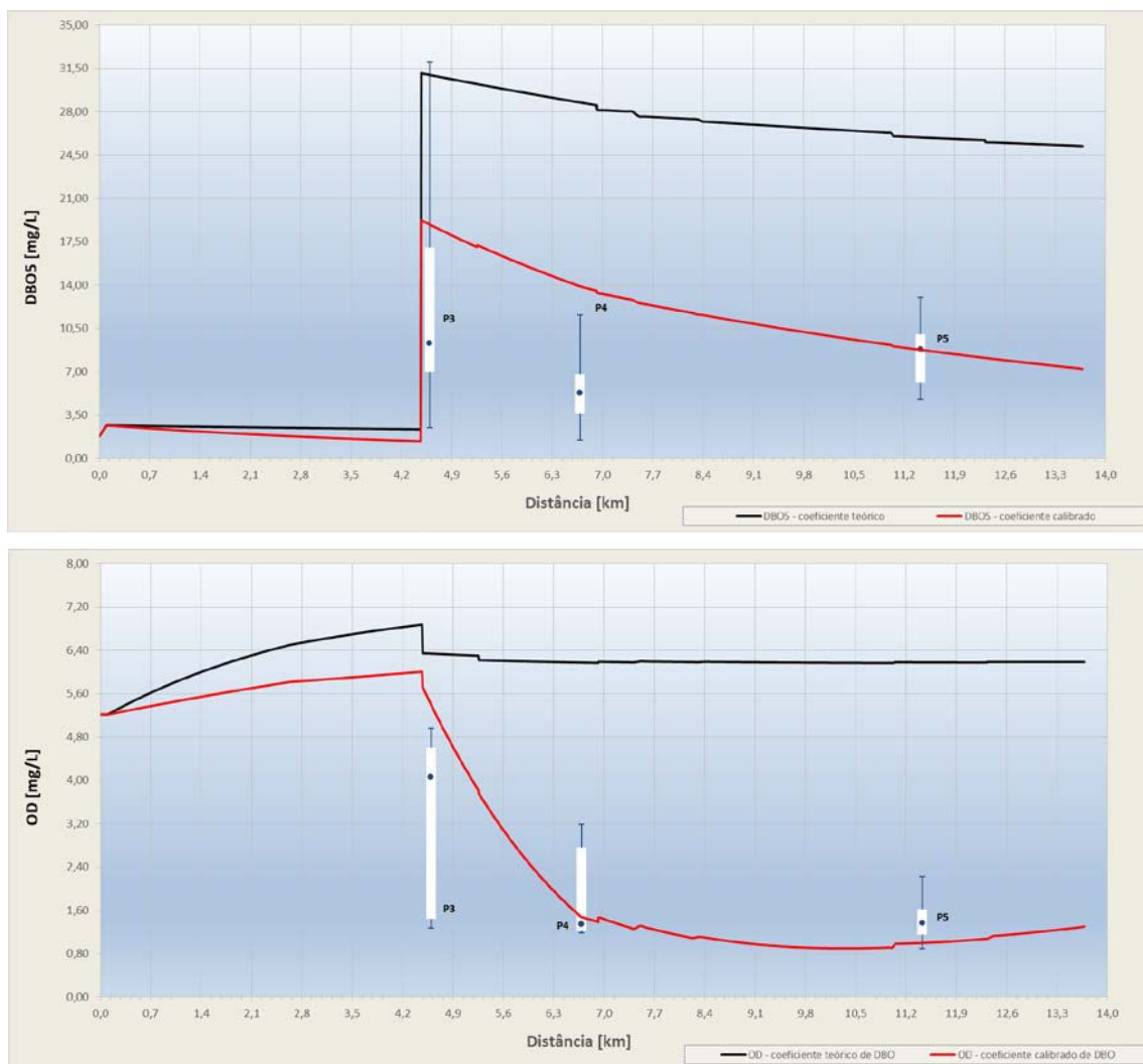
Figura 6: Perfis de concentração de \text{DBO}_5 e OD – coeficientes teórico e calibrado
