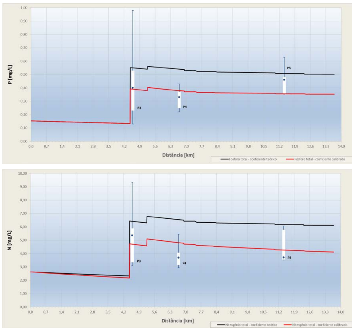
Figura 7: Perfis de concentração de fósforo total e nitrogênio total – coeficientes teórico e calibrado
