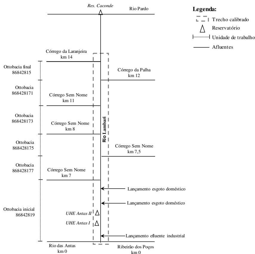
Figura 3: Diagrama unifilar do trecho calibrado do Rio Lambari
