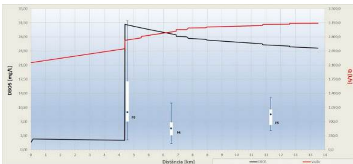
Figura 5: Perfis de vazão e de DBO 5 obtido no balanço hídrico, com os boxplots dos dados de campo, no trecho Rio Lambari
