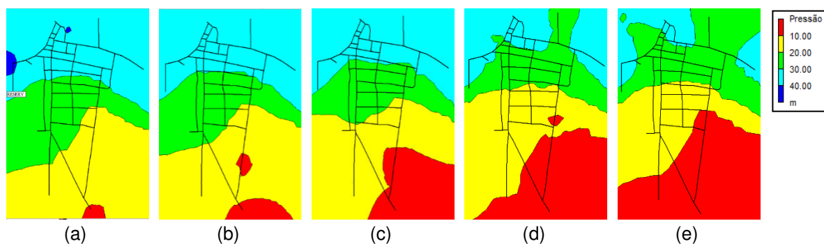
Figura 3 – Isolinhas de pressão da rede ampliada com acréscimos de vazão: (a) sem acréscimo, (b) acréscimo de 50%, (c) acréscimo de 100%, (d) acréscimo de 150% e (e) acréscimo de 170%.
