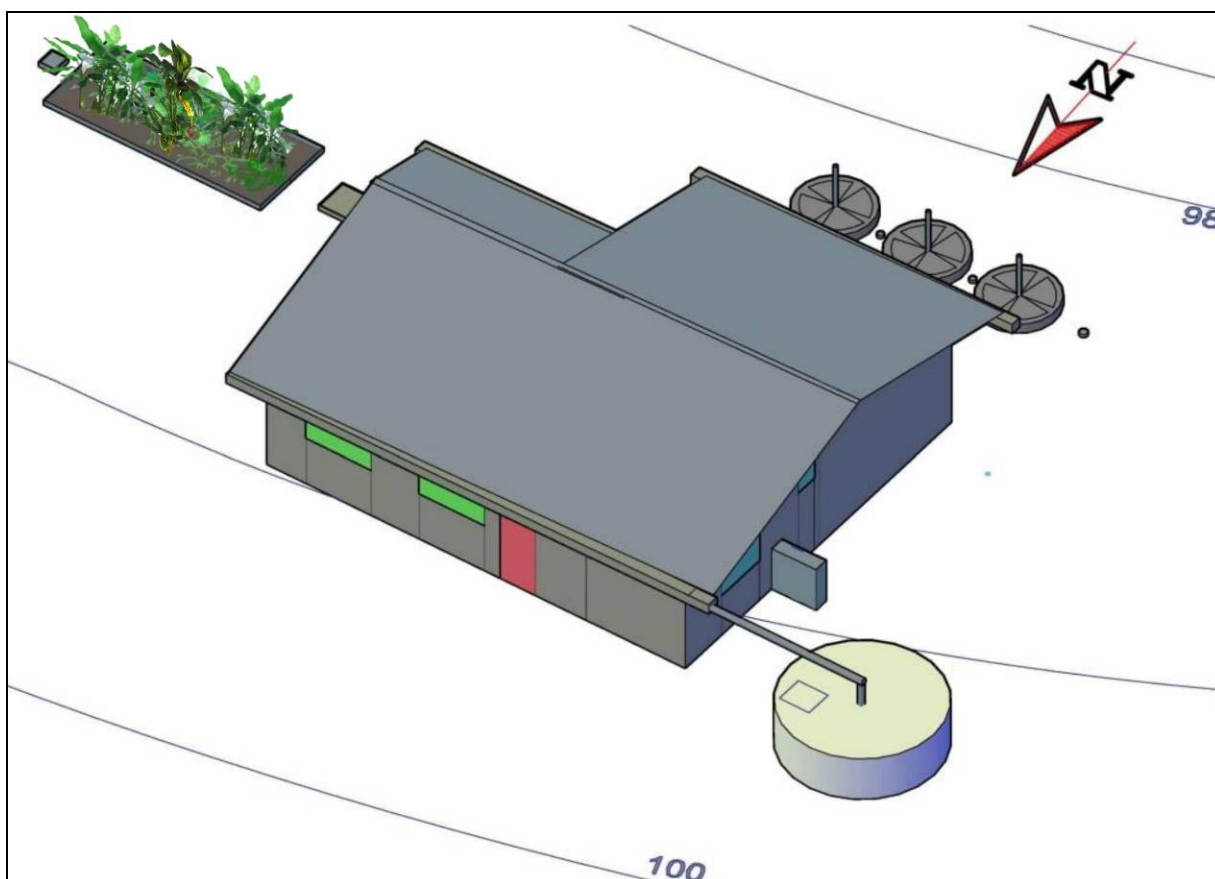
Figura 21: Layout do terreno com detalhes das tecnologias na visão da faixa da casa.
