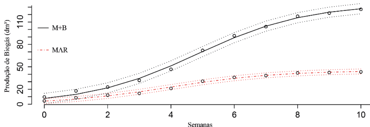
Figura 4. Curva ajustada do modelo Logístico ajustada ao volume de biogás acumulado para os tratamentos de maravalha + bagaço de cana (M+B) e cama de maravalha (MAR) com intervalos de confiança.
