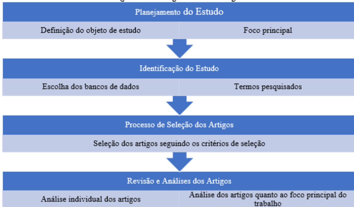
Figura 1 – Fluxograma Metodológico
