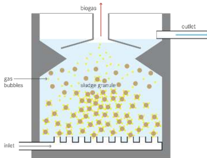
Figura 20 – Esquemática do UASB.
