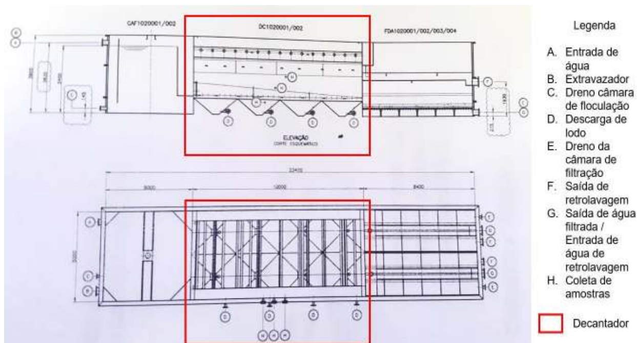
Figura 6 – Planta baixa da ETA convencional.
