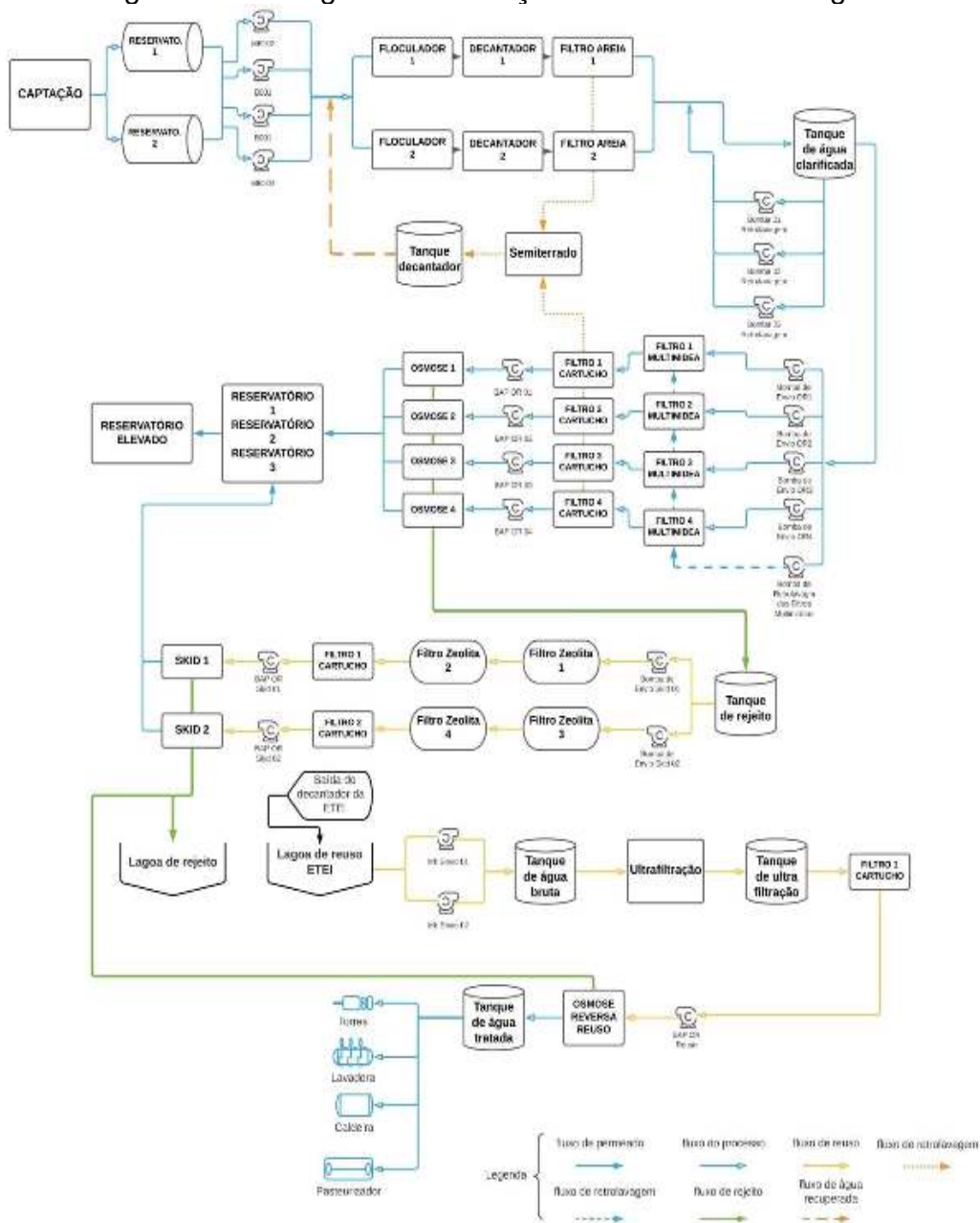
Figura 2 – Fluxograma da estação de tratamento de água.
