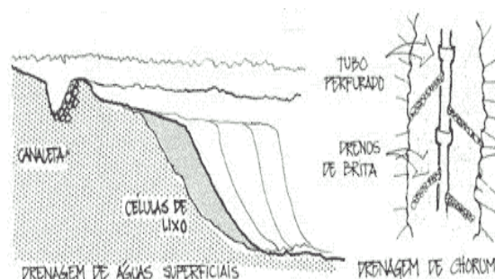
Figura 1- Esquema Aterro Delta 1 (Campinas-SP)
