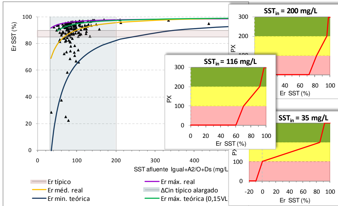
Figura 5 Curvas de Er_{SST} vs. C_{in} no tratamento secundário e funções de desempenho para três concentrações afluentes na gama 35-200 mg SST/L.
