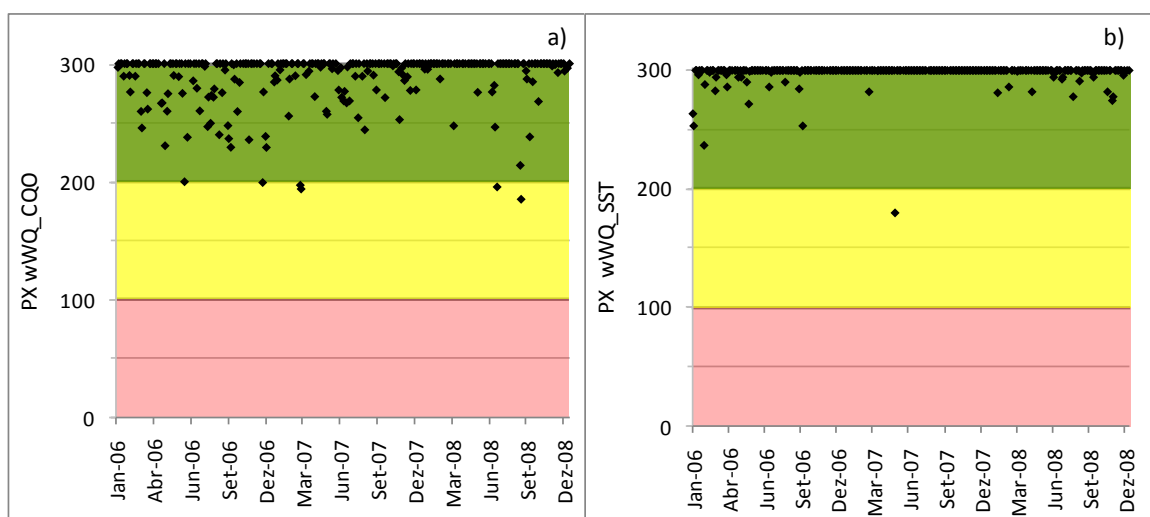
Figura 7 Índices de qualidade de água residual tratada para descarga: a) CQO e b) SST.
