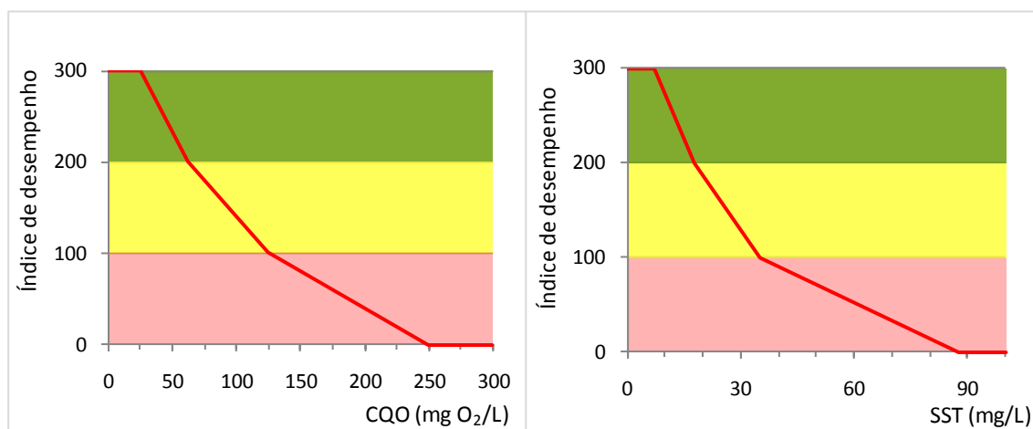
Figura 2 Funções de desempenho de Qualidade da água residual tratada para descarga segundo o DL 152/97.
