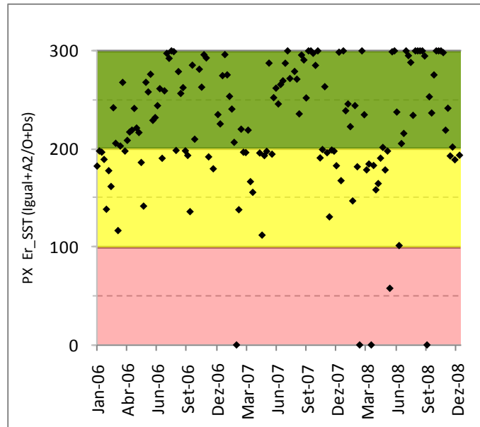
Figura 8 Índices de desempenho de eficiência de remoção de SST no tratamento secundário.
