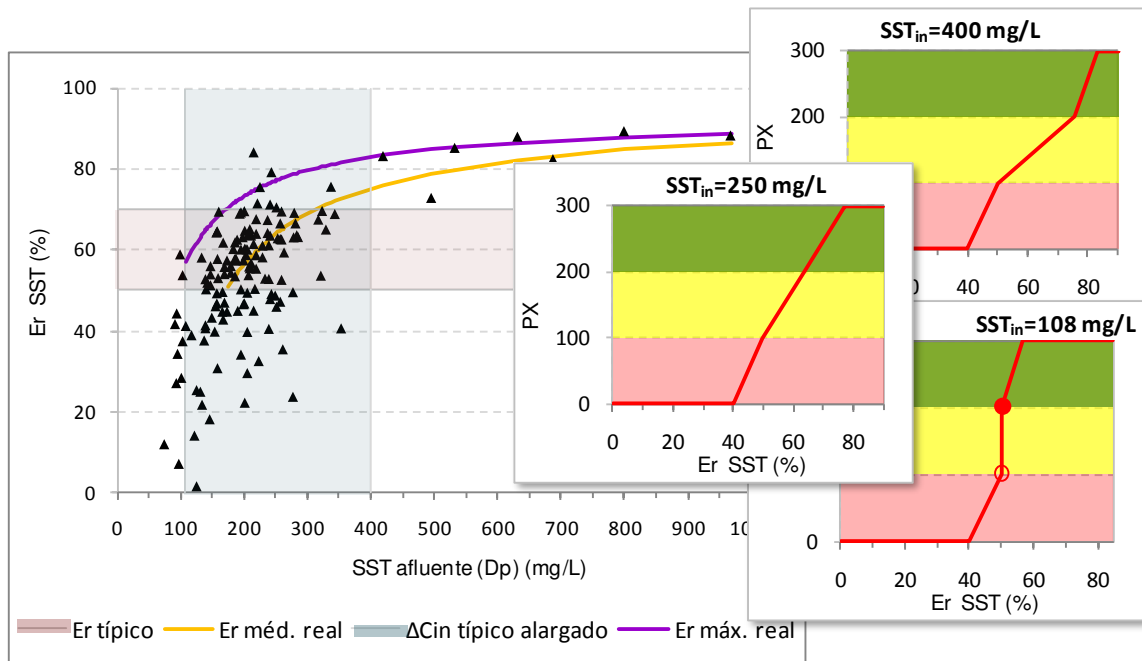
Figura 4 Curvas de Er_{SST} vs. C_{in} na decantação primária e funções de desempenho para concentração afluyente fraca, média e forte.
