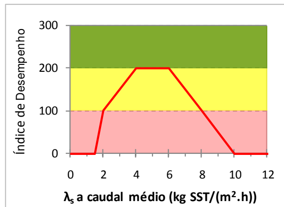
Figura 6 Função de desempenho para carga superficial de sólidos na decantação secundária.
