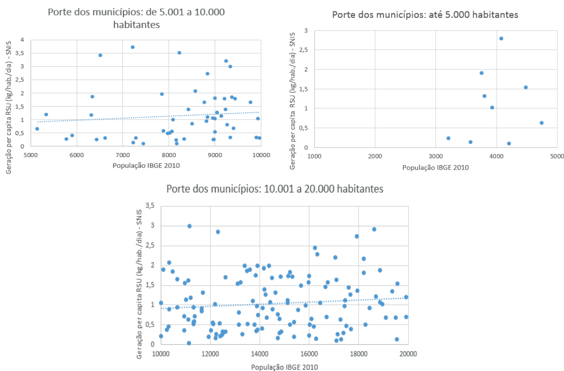
Figura 3 - Diagramas de dispersão municípios até 20.000 habitantes
