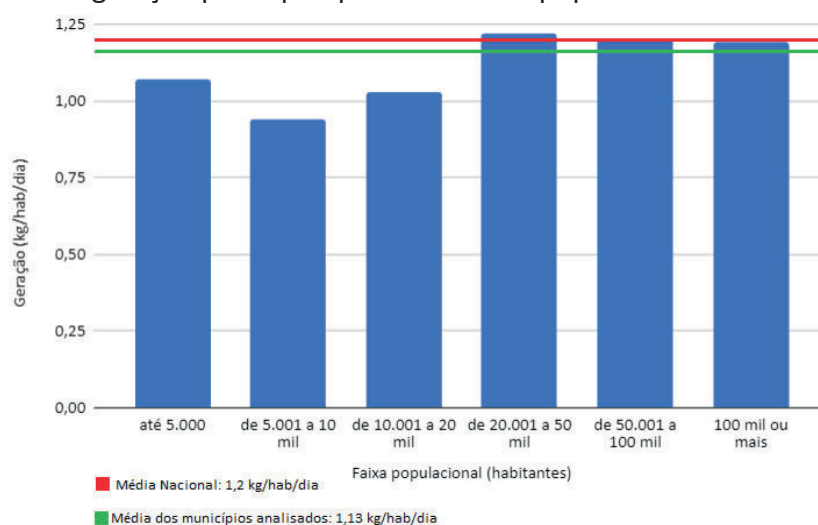
Figura 2 - Média da geração per capita para cada faixa populacional
